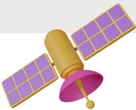
SATELITES
