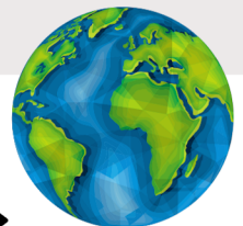
EARTH
